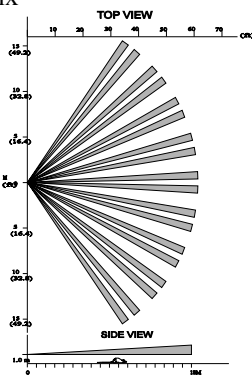
Рис 8 Диаграмма направленности линзы, обеспечивающей проход для животных
