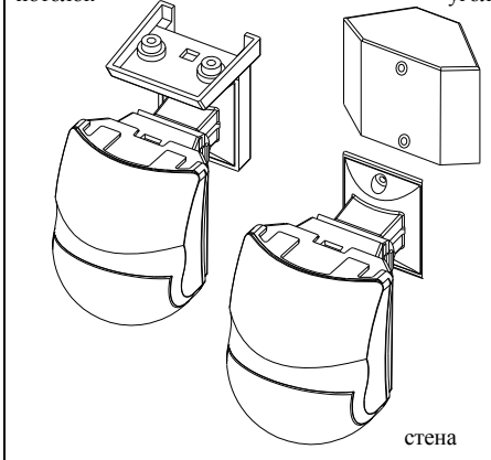
Рис 10 Варианты кронштейнов
